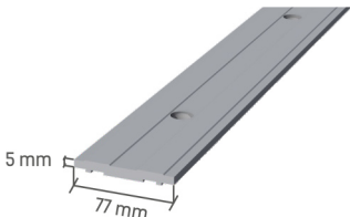
Profilo di allineamento e scolo acqua Codice / Code: GP Lunghezza / Length: 3-6 m
