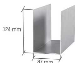
Profilo di contenimento In-floor base guide Codice / Code: LCO natural Lunghezza / Length: 3-6 m Solo per PP200 e PP400 Only for PP200 and PP400
