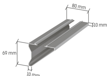
Carter inferiore Bottom cover Codice / Code: KI- NAT natural KI- ARG silver KI- INOX simil inox KI-9010 ral 9010 Lunghezza / length: 3-6 m
