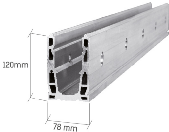
Profilo base intero forato Codice / Code: PL1 Lunghezza / Length: 3-6 m
