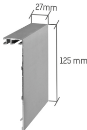
Carter laterale Codice / Code: KL- NAT natural KL- ARG silver KL- INOX simil inox KL-9010 ral 9010 Lunghezza / length: 3-6 m
