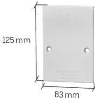
Tappo Codice / Code: T1- NAT natural T1- ARG silver T1- INOX simil inox T1-9010 ral 9010
