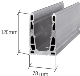
Profilo L 400 mm forato Codice / Code: PP400 Lunghezza / Length: 400 mm
