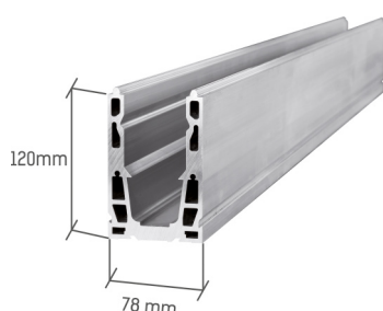
Profilo base intero forato Entire holed base profile Codice / Code: PL2 Lunghezza / Length: 3-6 m
