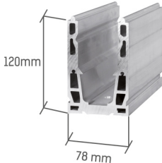
Profilo L 200 mm forato Codice / Code: PP200 Lunghezza / Length: 200 mm
