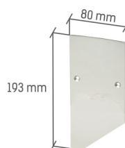
Tappo per carter inferiore End cap for bottom cover Codice / Code: T3- NAT natural T3- ARG silver T3- INOX simil inox T3-9010 ral 9010
